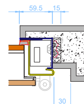
Controtelaio BLITZ.
