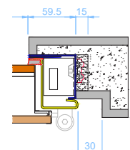
Controtelaio BLITZ.
